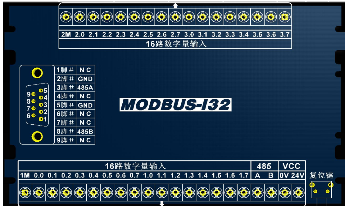
MODBUS-I32
