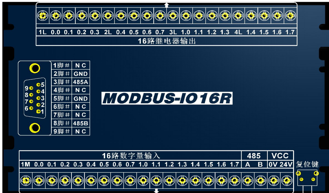
MODBUS-IO16R
