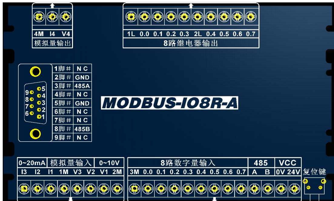
MODBUS-I08R-A
